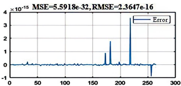
Fig. 24 Error test data ( \phi parameter)
